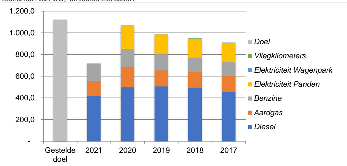
Figuur 3. Vergelijking van ton CO 2 -emissie tussen 2017 t/m 2020 & 2021 per energiestroom en het gestelde (reductie)doel van 1.121,9 ton CO 2 voor de totale emissie in het jaar 2021.
